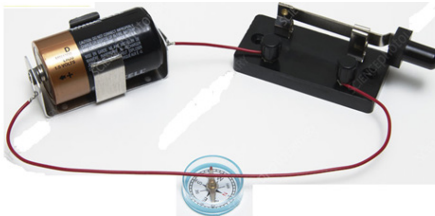
ስዕል 2.39 መግነጢሳዊ መስክ የኤሌክትሪክ ኻረት በተሸከመ ቀጥ ያለ ሽቦ
