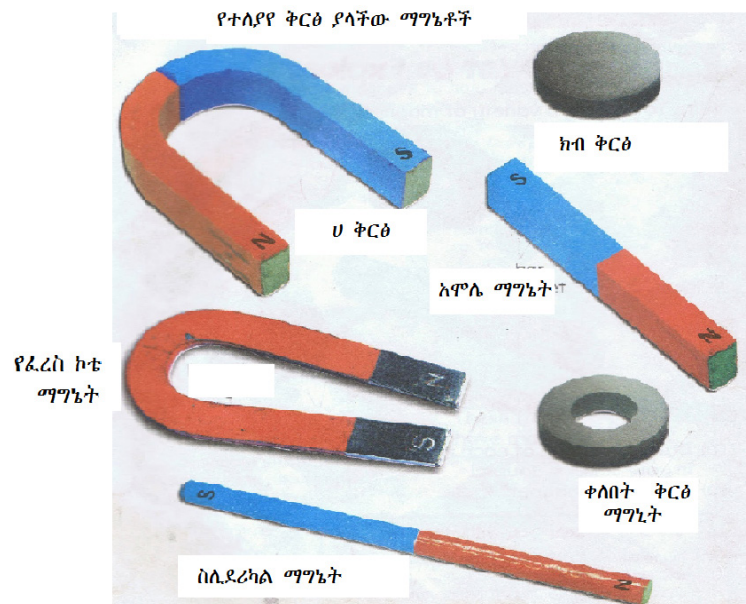
ስዕል 2.36 የተለያዩ ቅርፅ ያላቸው ማግኔቶች
