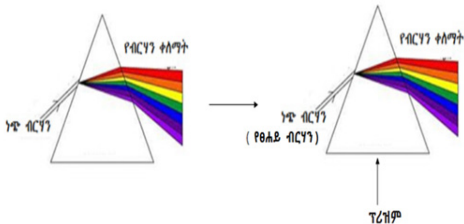
ስዕል 2.27 የብርሃን መበተን
