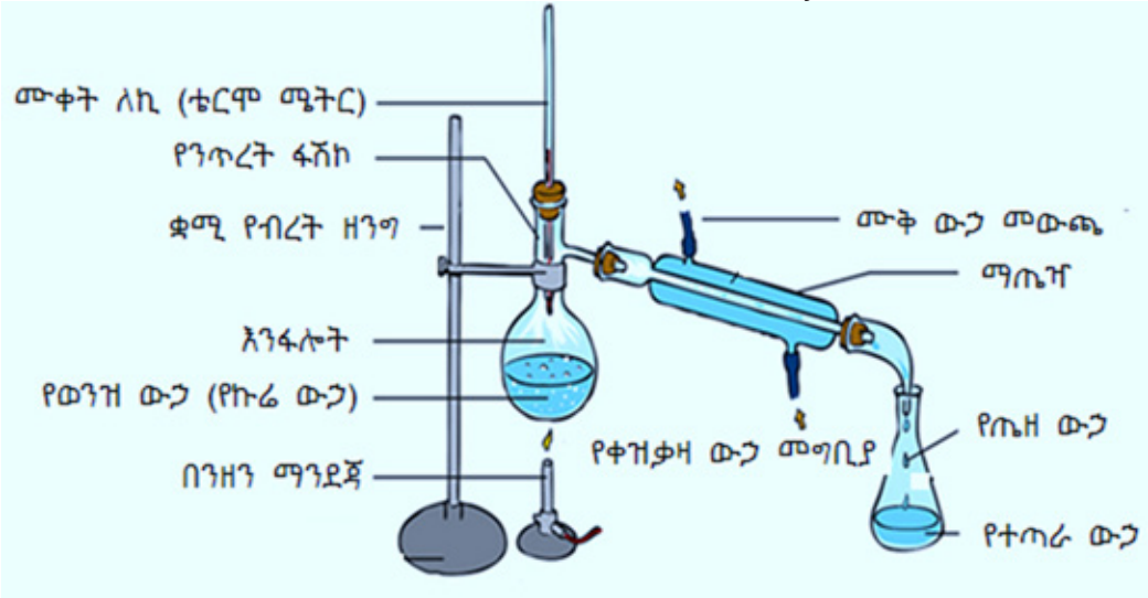
ስዕል 2.8 የንጥረት መሳሪያ ቅንብር
