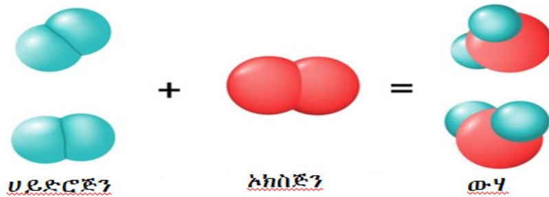
ስዕል 2.3 የወደር ወይም የንፅፅር ጽንሰ ሃሳብ በኬሚካዊ ፅግበራ
