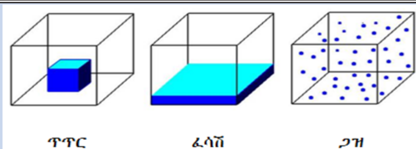
ስዕል 2.12 የቁሶች ሁነቶችን ቅርፅ እና ይዘትን ማነፃፀር
