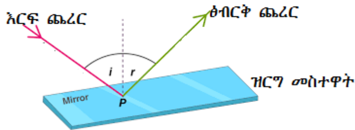
ስዕል 2.23 የብርሃን ፅብረቃ
