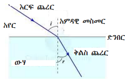
ስዕል 2.24 የብርሃን መቀለስ
